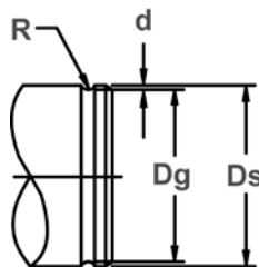
軸径 & 溝寸法
