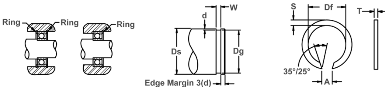
軸径 & 溝寸法
